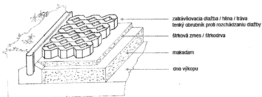
Schéma konštrukčného riešenia odstavnej plochy na zatrávňovacej dlažbe
